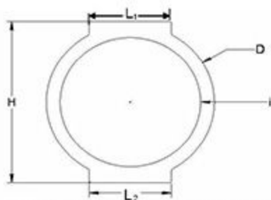
KOLLEKTÖR ÜRETİM ÖLÇÜ VE TOLERANSLARI
